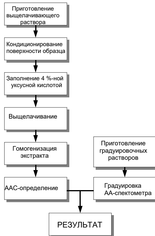
Рисунок А5.1: Методика определения выщелачиваемого металла
