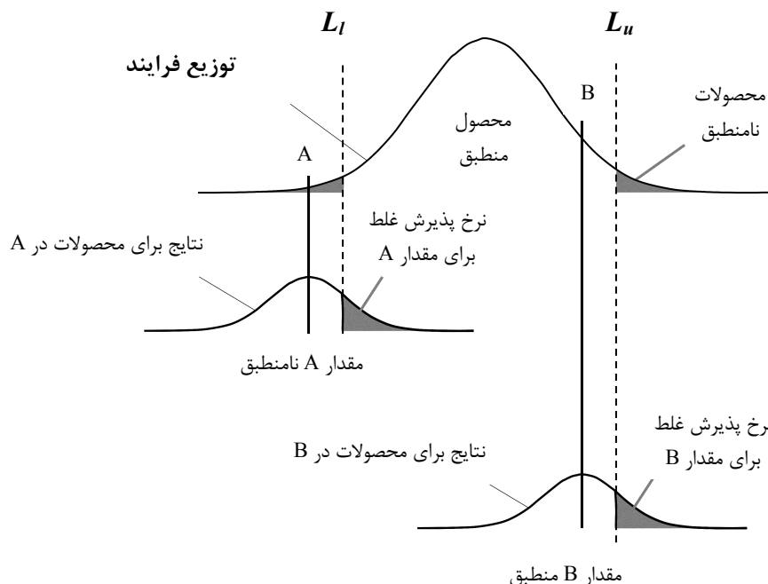
شکل ۶- ریسک تولیدکننده و مصرف‌کننده. شکل بالا توزیع مقادیر اندازه‌دهنده به دست آمده در فرایند تولید یا دیگر فرایندها را نشان می‌دهد. گستره مجاز بین حدود L_l و L_u و توزیع مقادیر اندازه‌گیری شده ارقام آزمون در A و B نیز نشان داده شده است. برای جزئیات بیشتر متن را بخوانید.
